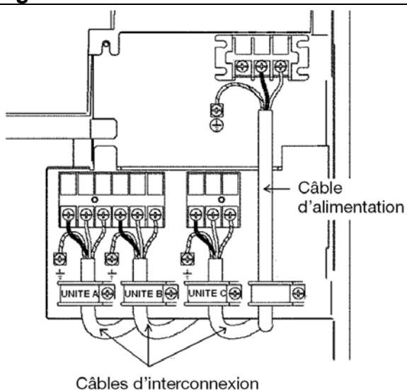
Schéma de câblage des unités intérieures sur l'unité extérieure
